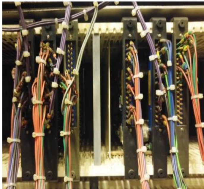
Szekrény belső vezetékvezése
