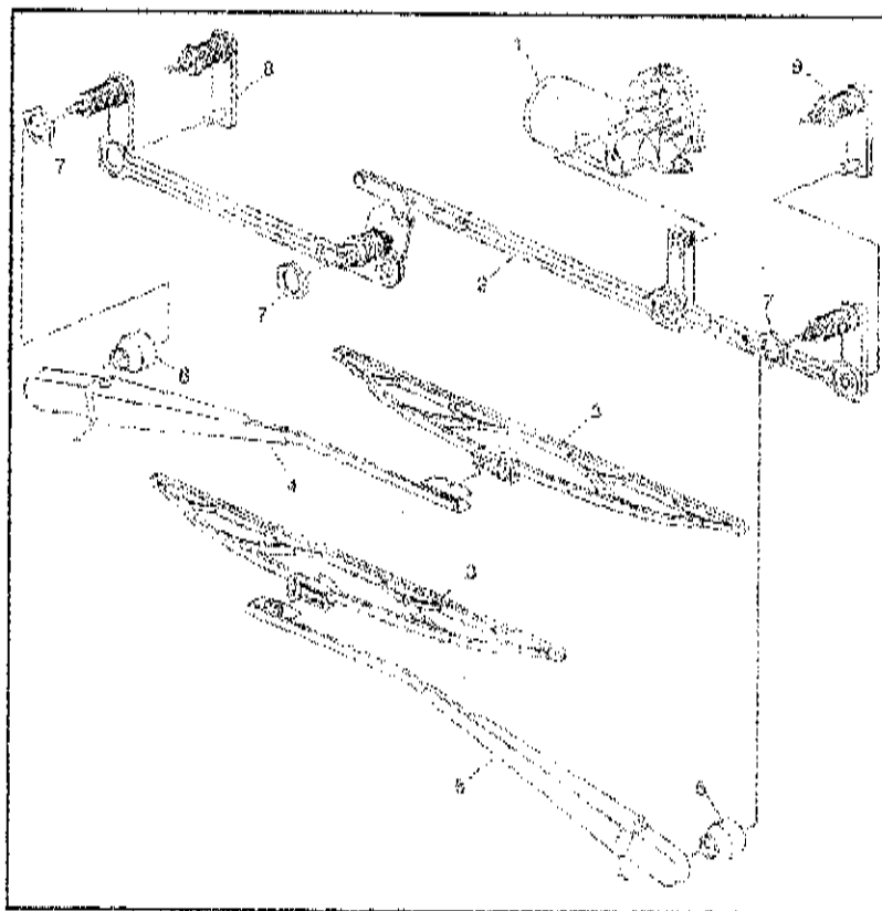
FIG. 1005 Ablaktörők
